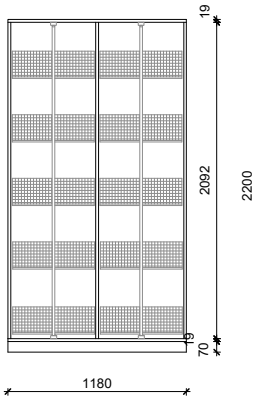
00.16.01 Apothekerschrank Innenaufteilung
